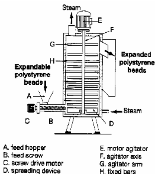
شکل ۲-۵- پیش منبسط کننده پیوسته
