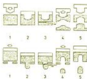
شکل ۲-۱۵- ایجاد اشکال مختلف با استفاده از اعمال فشار، قالب و برش
