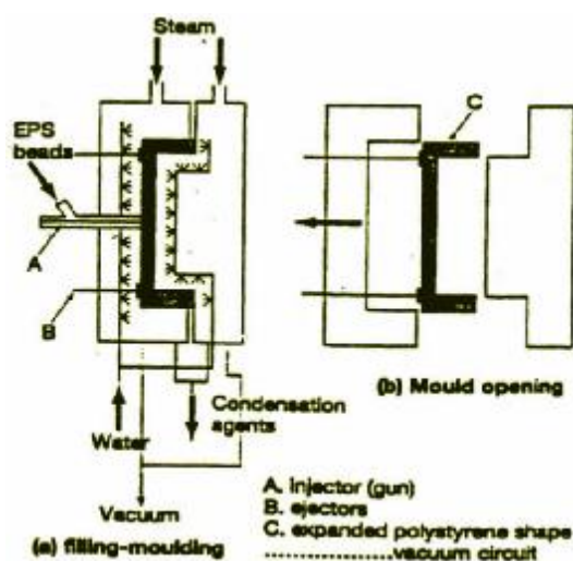
شکل ۲-۱۲- قالبگیری شکلی پلی استایرن منبسط شده
