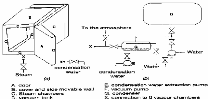
شکل ۲-۸- تجهیزات خلاء و قالب بلوک EPS
