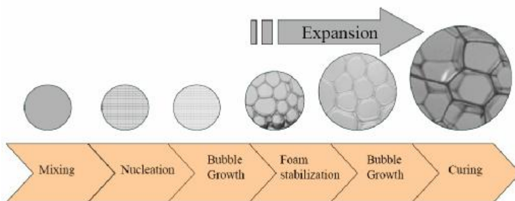
شکل ۲-۲- فازهای مختلف فوم شدن
