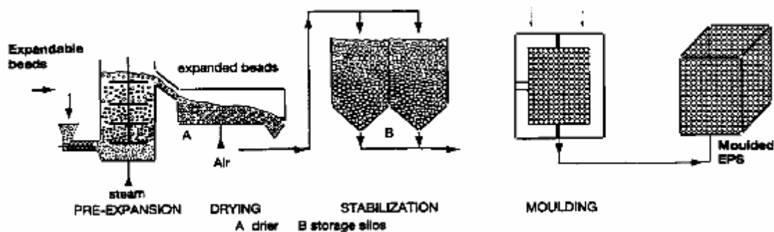
شکل ۲-۴- فرآیند تولید
