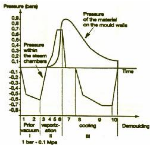
شکل ۲-۱۱- مراحل قالبگیری بلوک پلی استایرن انبساطی
