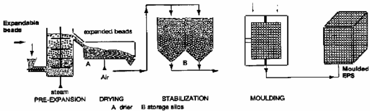
شکل ۲-۲- فرآیند تولید
