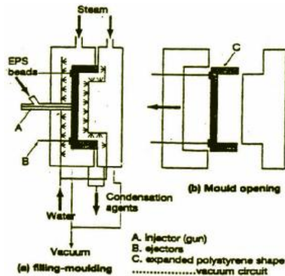
شکل ۲-۵- قالبگیری شکلی پلی استایرن منبسط شده
