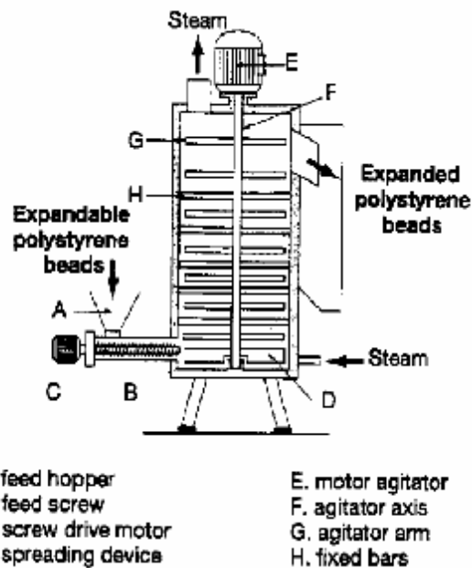
شکل ۲-۳- پیش منبسط کننده پیوسته
